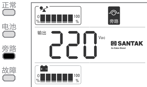
(旁路工作模式)
