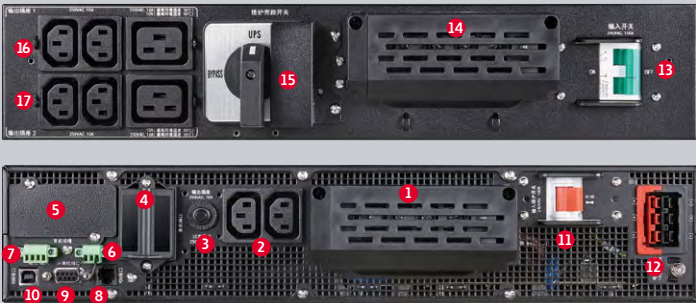
6-10K手动维修旁路及智能配电单元
