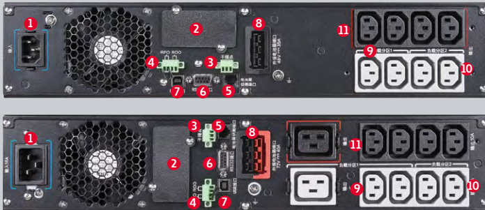
PT1K后面板接口
