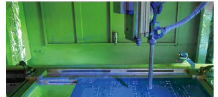
PCBA喷涂后蓝光检测
