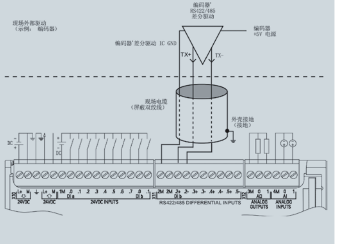
差分输入示意图
