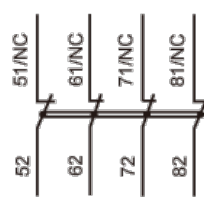
4NC(LAEN04)
