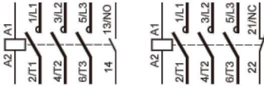
1NO+1NC(LANN11)
