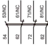
1NO+3NC(LANN13)
